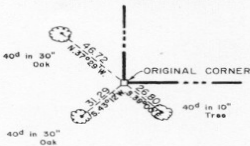
S.W. CORNER
