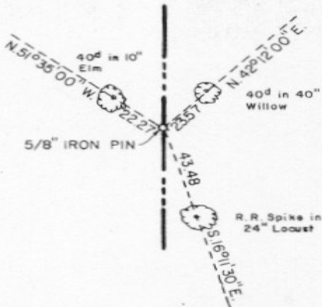
S.W. CORNER
