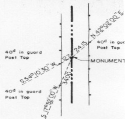
S.E. CORNER
