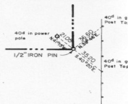
S.E. CORNER
