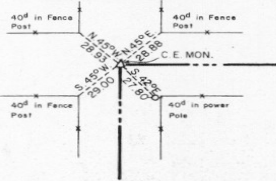
N.W. CORNER
