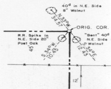
N.E. CORNER
