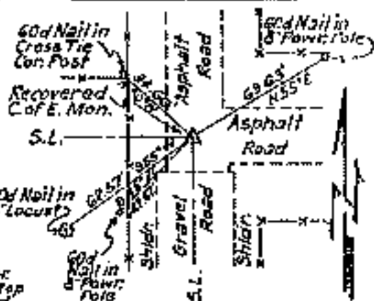
N.E. CORNER
