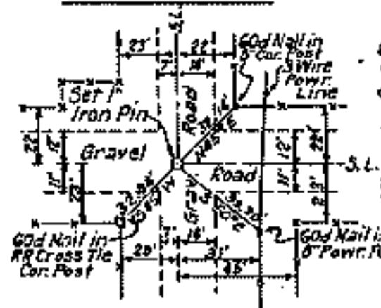
S.W. CORNER
