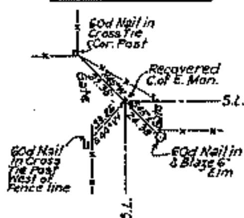
N.W. CORNER
