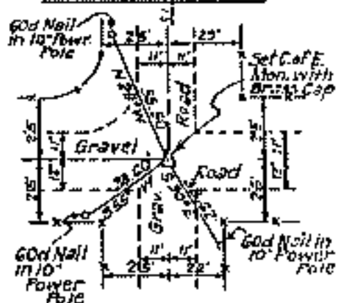
S.E. CORNER
