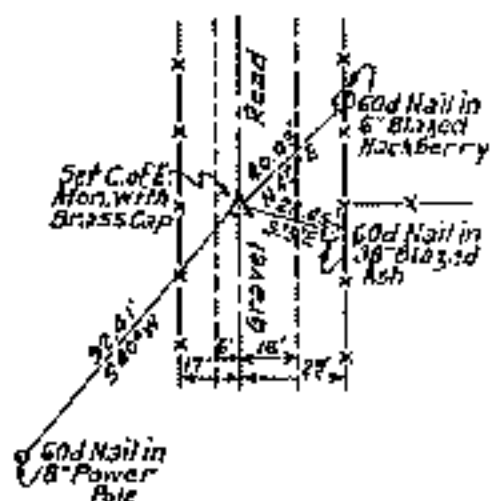
S.E. CORNER
