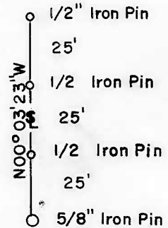
S.E. CORNER
