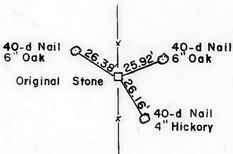
S.W. CORNER
