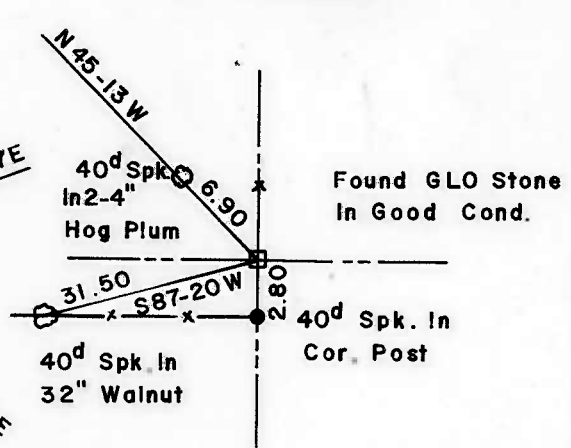
SE. CORNER
