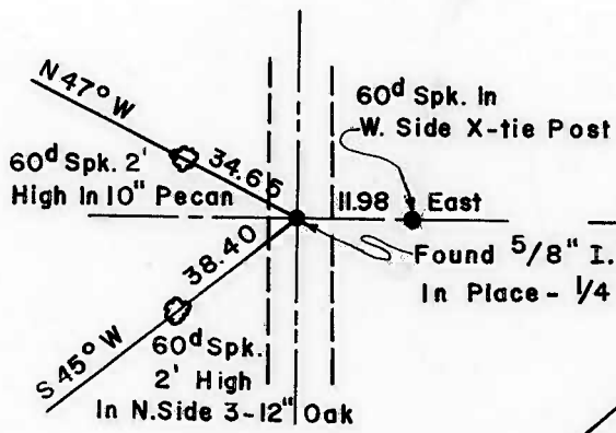
S.W. CORNER
