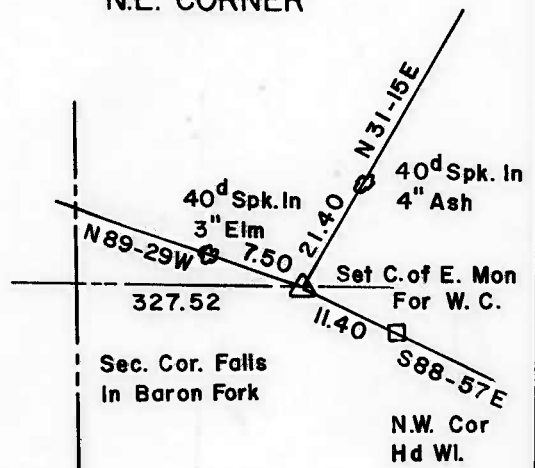
N.E. CORNER
