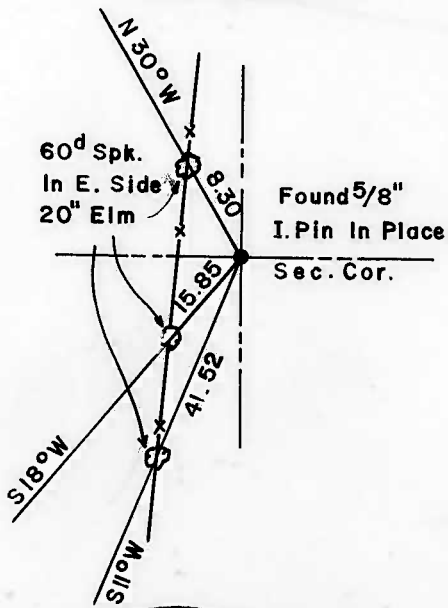
S.W. CORNER
